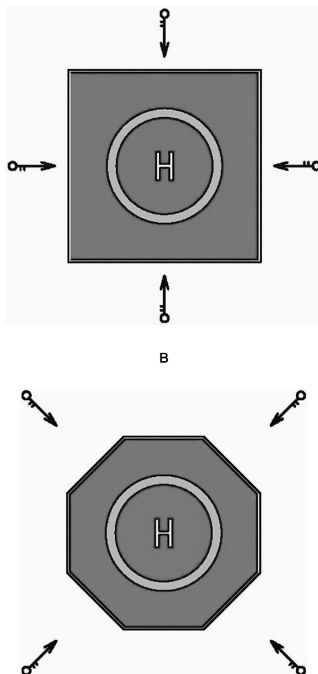
Рисунок А.1 - Схемы размещения стационарных лафетных стволов
