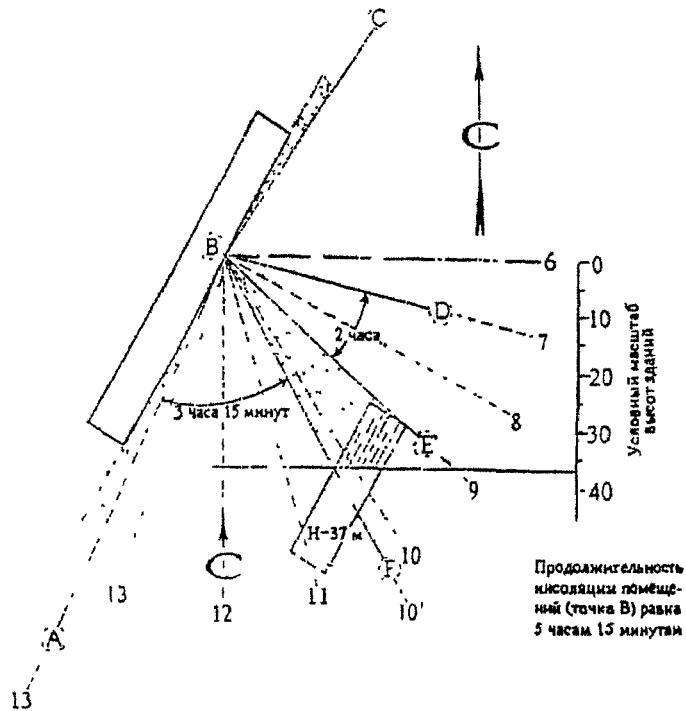
Рис. 5. Схема определения инсоляции.
