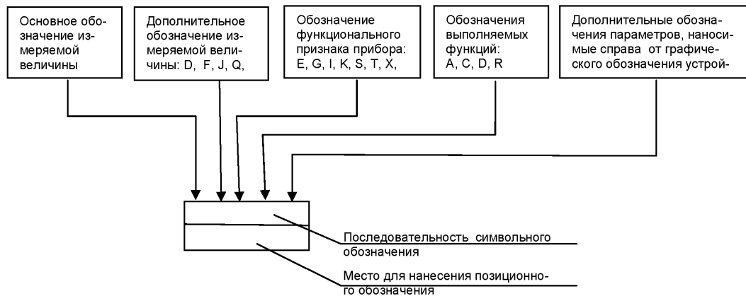
Рисунок 1. Принцип построения условного обозначения прибора
