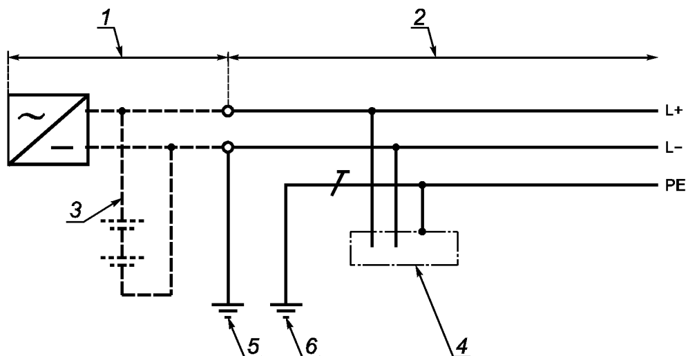
Тип b) - трехпроводная система
