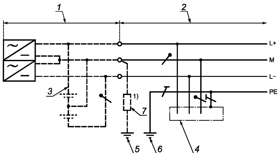
Тип b) - трехпроводная система
