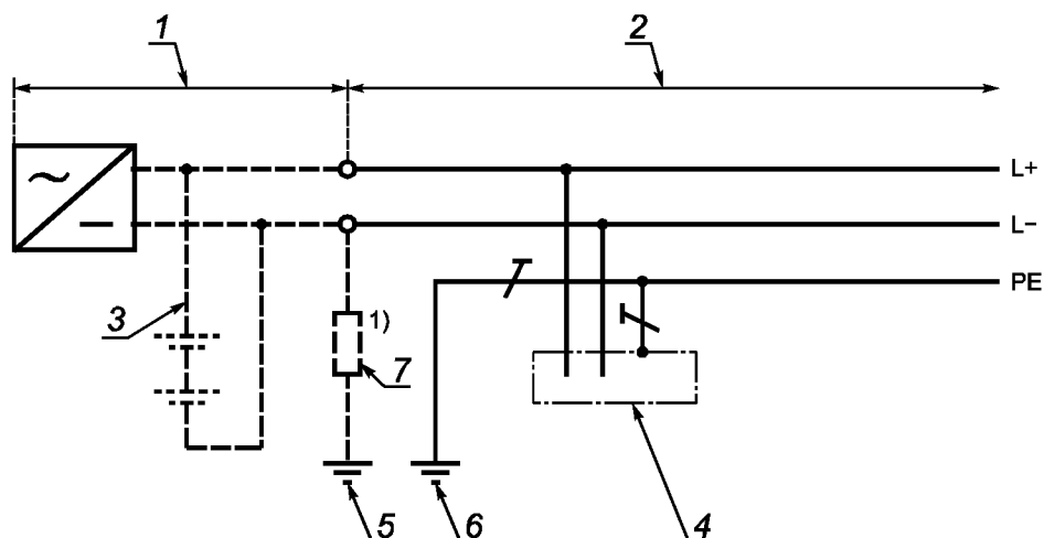
Тип b) - трехпроводная система
