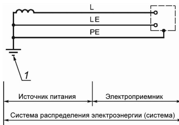
1 - заземляющее устройство источника питания
