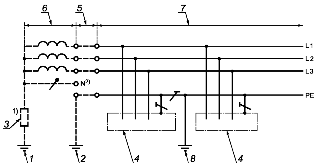
1 - заземление источника питания; 2 - защитное заземление системы; 3 - полное сопротивление; 4 - открытые проводящие части; 5 - распределительная электрическая сеть (при ее наличии); 6 - источник питания; 7 - электроустановка; 8 - защитное заземление в электроустановке
