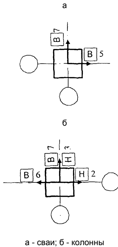
Рисунок 3. Примеры указания действительных отклонений осей элементов от разбивочных осей на плане
