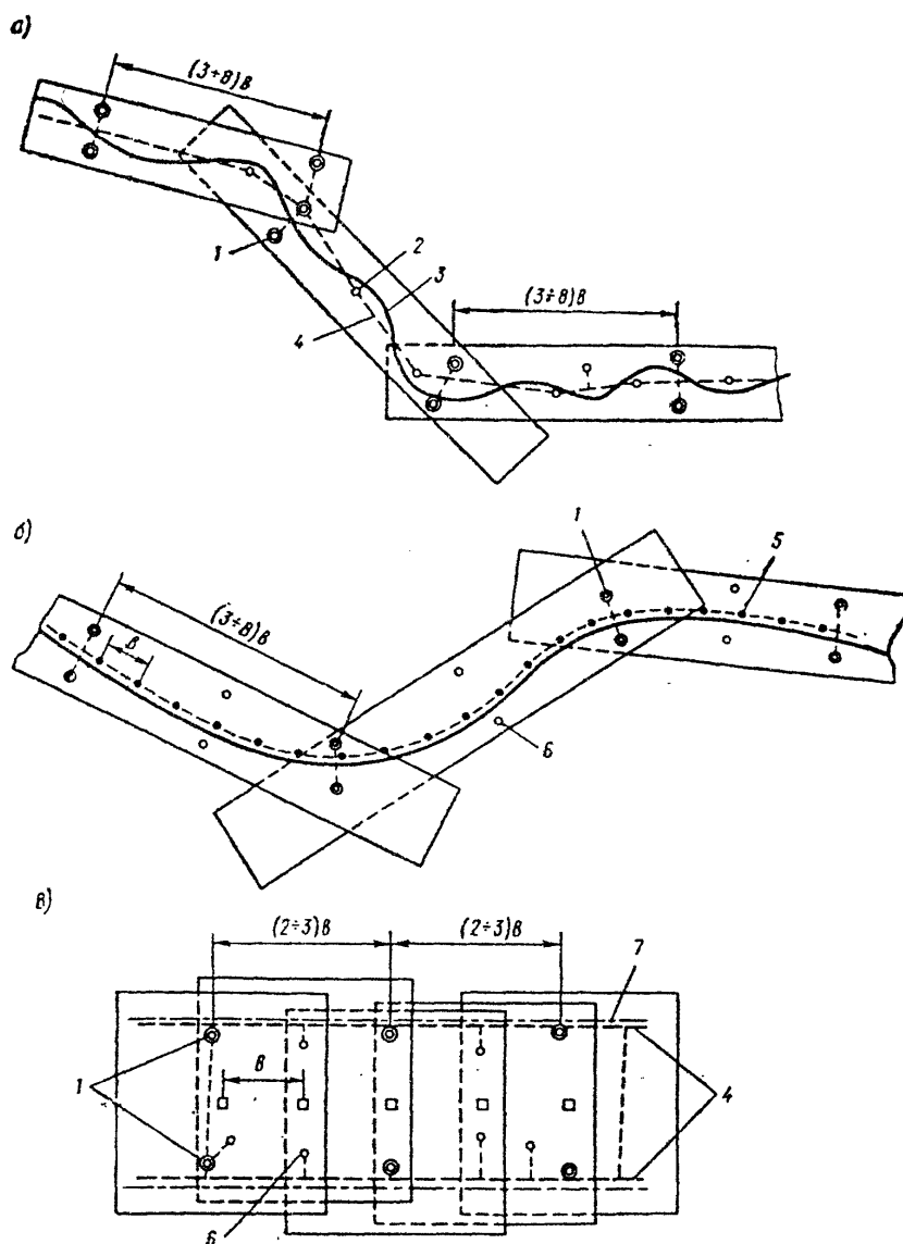
Рис. 1. Схема расположения опознаков для обоснования маршрутов аэрофотосъемки при изысканиях а - новых линий; б - вторых путей; в - для усиления и реконструкции больших станций и узлов; 1 - планово-высотные опознаки; 2 - высотные опознаки; 3 - трасса; 4 - магистральный ход; 5 - точки на земляном полотне, привязанные к пикетажу; 6 - контрольные точки; 7 - границы рабочей площади
