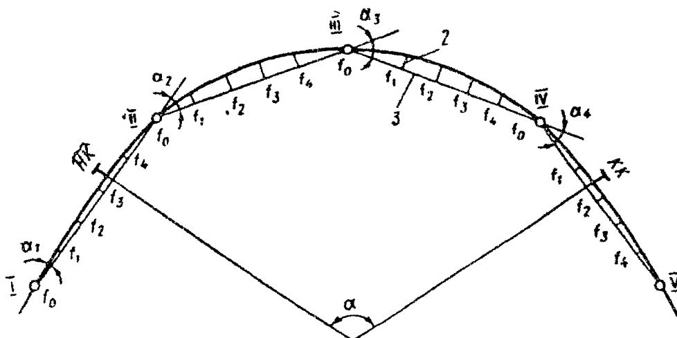
Рис. 2. Схема съемки кривых методом И.В. Гоникберга: I - V - стоянки теодолита; 1 - наружный рельс;
