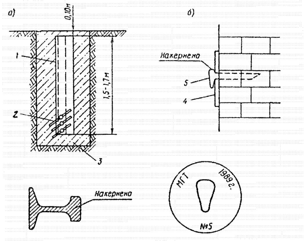
Рис. 2. Образец закрепления точек базисного и магистрального ходов грунтовыми и стенными знаками: а - рельсовые рубки; б - костыли; 1 - рельс; 2 - металлические штыри; 3 - щебень, песок; 4 - металлическая пластина; 5 - костыль
